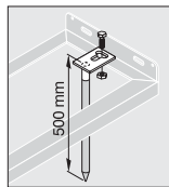
Bodenanker (2er-Set) Art-Nr. 105 003
