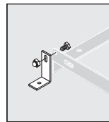
Bodenmontage-Winkel (2er-Set) Art.-Nr. 105 002
