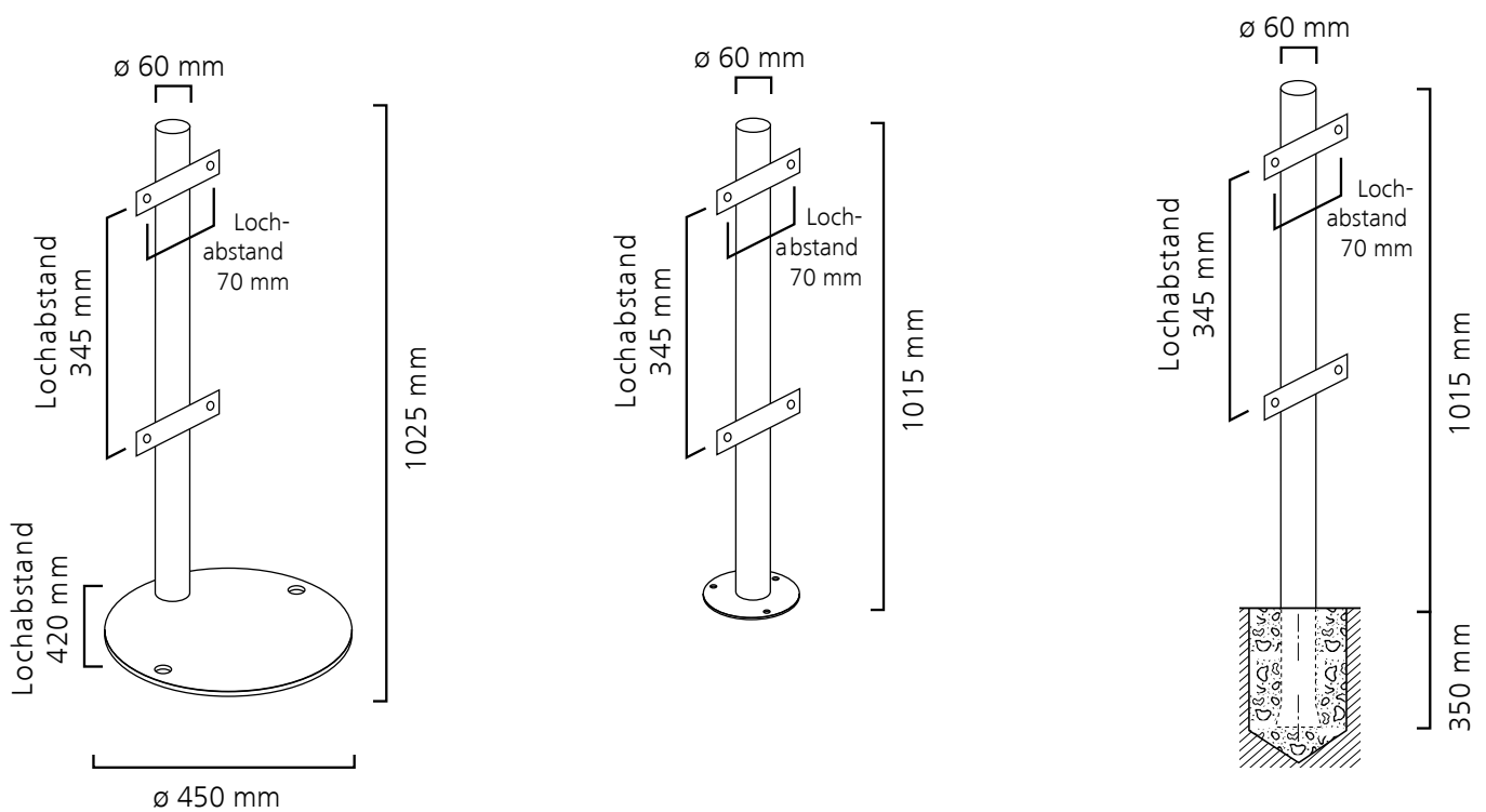
Standrohr mit Flansch
